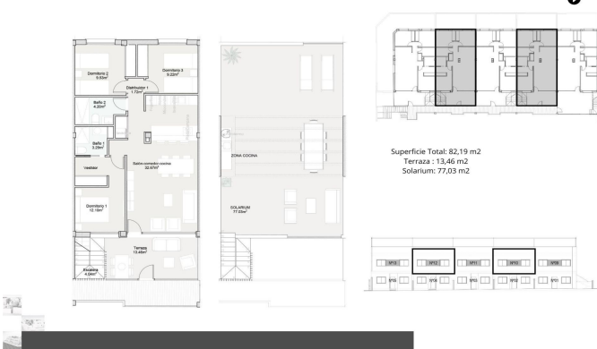
VIVIENDA TIPO Nº10 Y 12 - 3 DORMITORIOS
