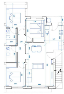
PLANTA BAJA (91,10 m2)
