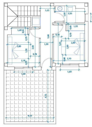
PLANTA PRIMERA
